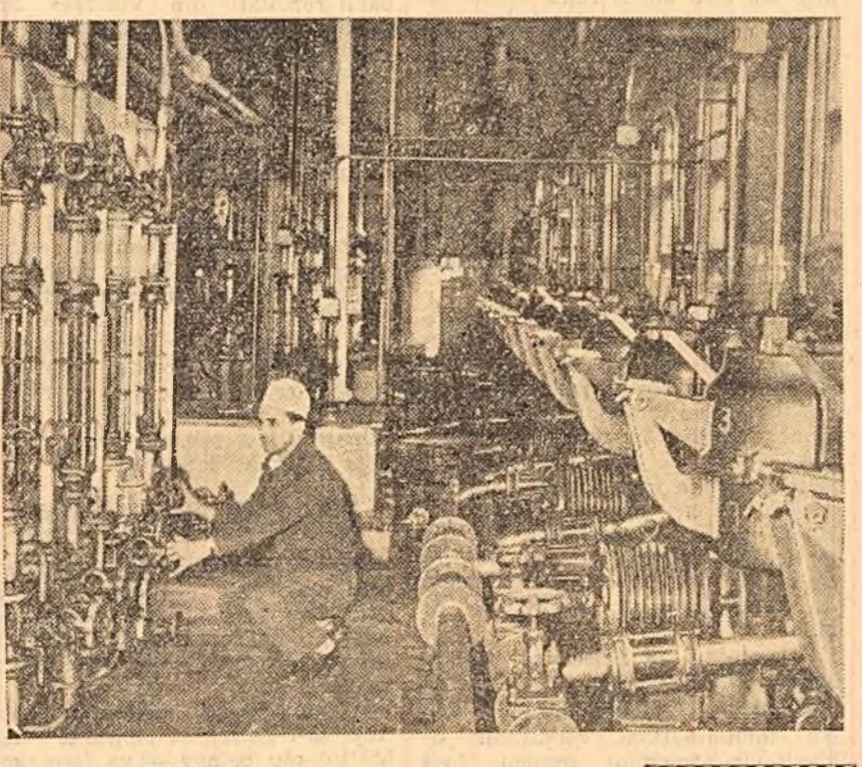
Fabrica de antibiotice din Iași este dotată cu utilaj modern, necesar producerii penicilinei. Iată-l pe lăcătușul Manolo Apostol, supraveghînd funcționarea unui rotametr, care indică intrarea lichidului de cultură în emulgatoare. (Foto Gh. Vințilă)
