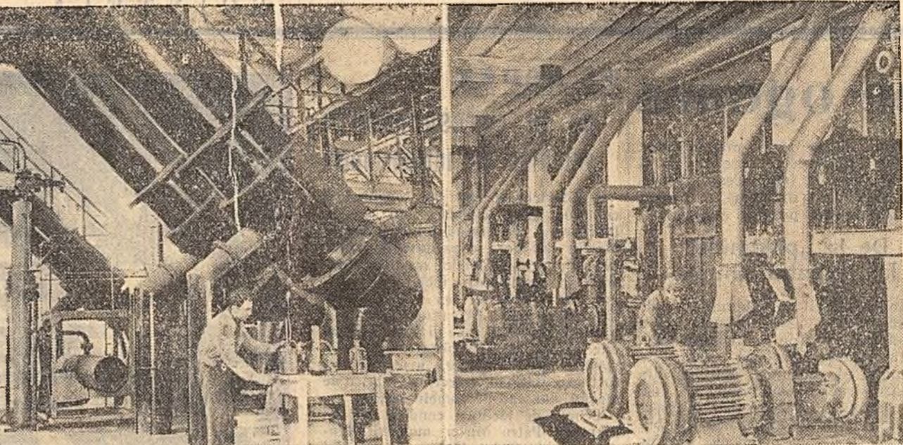
Fotografiile de mai sus înfățișează două aspecte de la uzina chimică Năvodari: instalația de prăjire a sărului în strat fluidizant (stînga), și instalația de circulație a acizilor, la linia de acid sulfuric. (Foto R. Costin)
