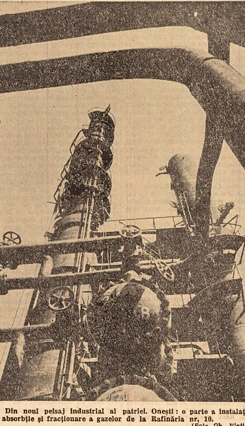
Din noul peisaj industrial al patriei. Onești: o parte a instalației de absorbție și fracționare a gazelor de la Rafinăria nr. 10. (Foto Gh. Vințilă)
