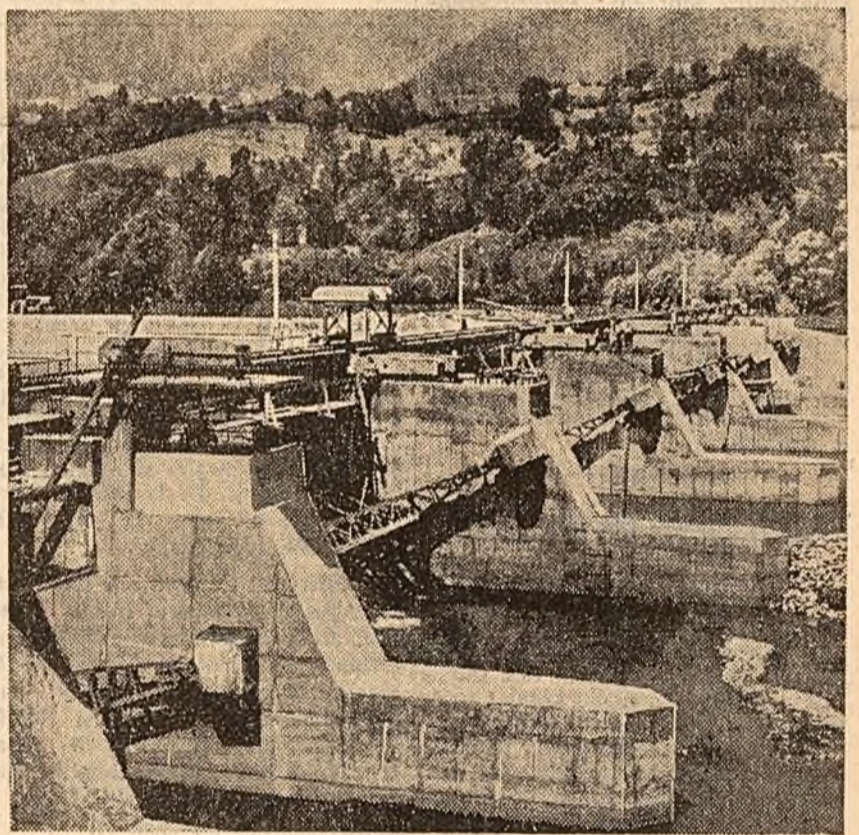
De curînd a fost dat în funcțiune barajul destinat captării apei de răcire pentru centrala termoelectrică Paroșeni.
