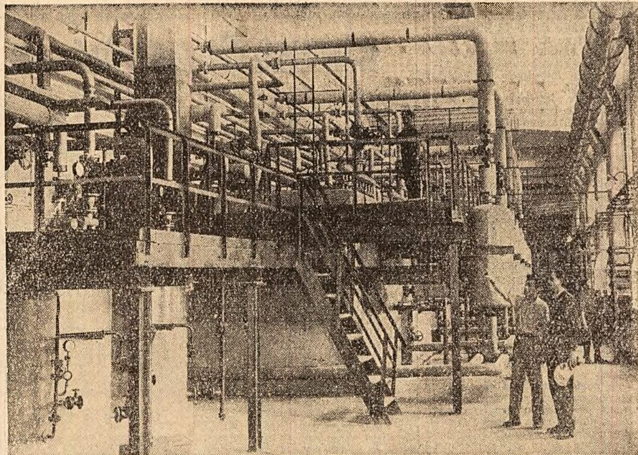
Instalația de lichefiere a clorului din cadrul Combinatului chimic Borzești.
