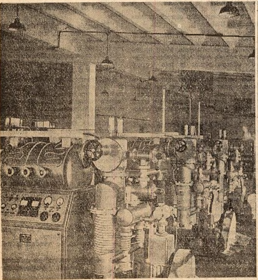
În secția de nichelare a uzinelor „Grigore Preoteasa” din Capitală. În fotografia din stânga: mașina de depunere în vid a bismutului și selenului pentru fabricarea plăcilor redresoare. În fotografia din dreapta: baia rotativă de nichelare.
