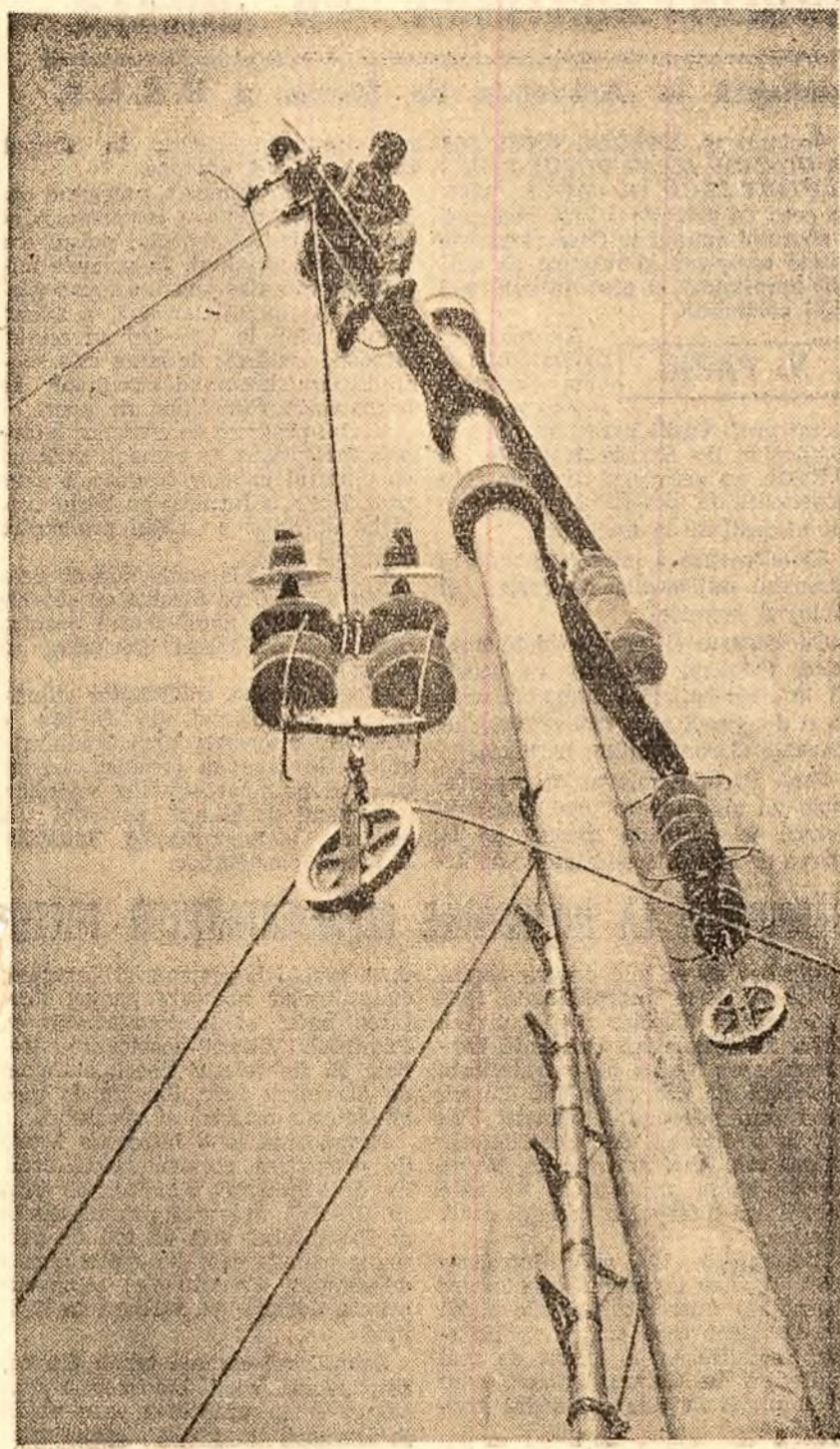
Curind o noua linie electrica va fi data in folosinta. In fotografia se monteaza izolatori la linia de 80 kW, Budesti-Olteni, linie care va imbunatati aprovizionarea cu energie electrica a acestei parti a tarii. (Foto: Agerpres)
