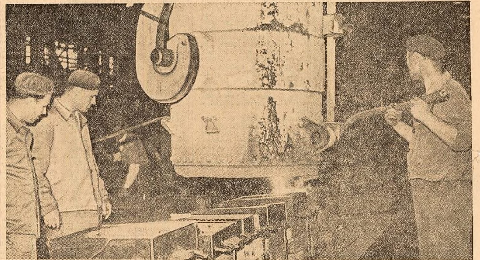
La uzinele „23 August” din Capitală unul din procedeele tehnologice moderne aplicate în turnătorie este turnarea în cochile. Prin acest procedeu se reduce consumul de metal lichid la maselote cu 30 la sută, piesele au o suprafață curată, se reduce adăosul de prelucrare cu 5 la sută și rebuturile. În fotografie: Dumitru Dinulescu, șef de echipă, Mihai Ciocan, turnător, și manipulantul Ion Rusu în timpul operației de turnare în cochile. (Foto: M. Cioe)
