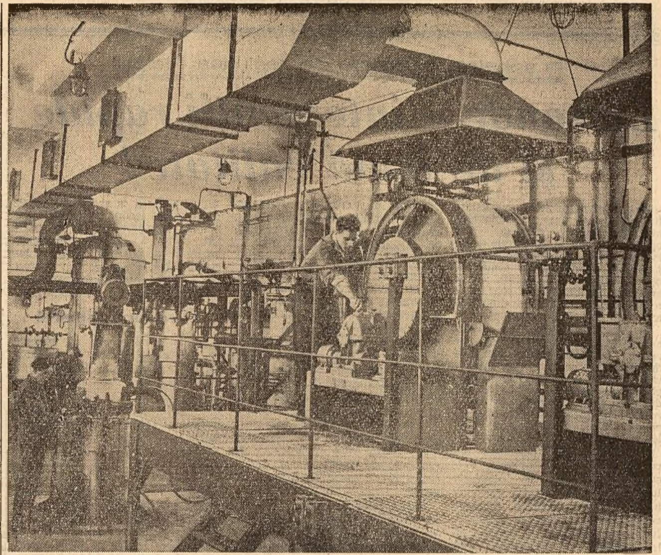
Aspect din hala de sinteză a nitrului acrilic de la stația-pilot a fabricii de fire și fibre sintetice Săvinești. (Foto R. Costin)
