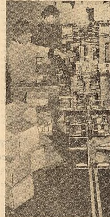
Mașina automată pentru ambalarea filmelor „Leika” la fabrica de filme „Agfa” din Wolfen (R.D.G.).
