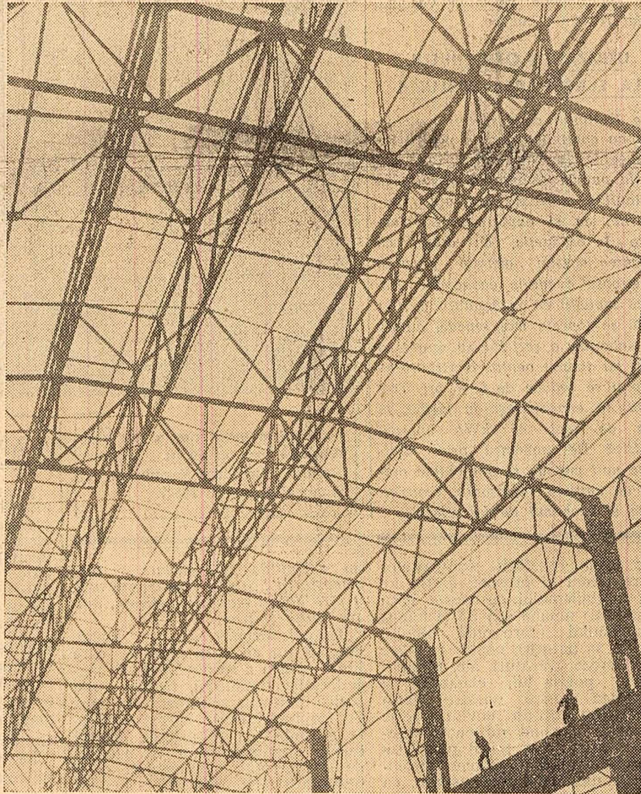
Cînd în decembrie 1960 se punea primul stîlp pe fundație, era greu să-ți închipui că, după un an, noile laminare ale Hunedoarei vor lua asemenea proporții încît să nu le poți cuprinde dintr-o singură privire. Iată, în fotografie, construcția metalică a halelor laminatoarelor care avansează cu fiecare zi.
