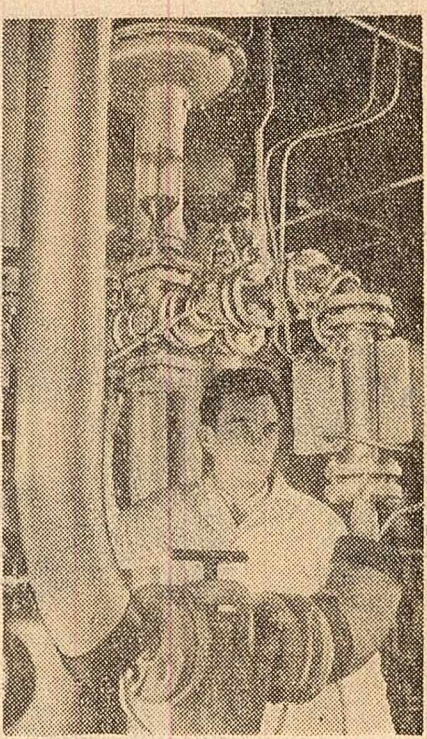
In secția de acizi grași a fabricii de produse chimice de sinteză organică „S.I.N.” din Capitală se urmărește debitul de alimentare la instalația de distilare a acizilor grași sintetici. (Foto: Agerpres)
