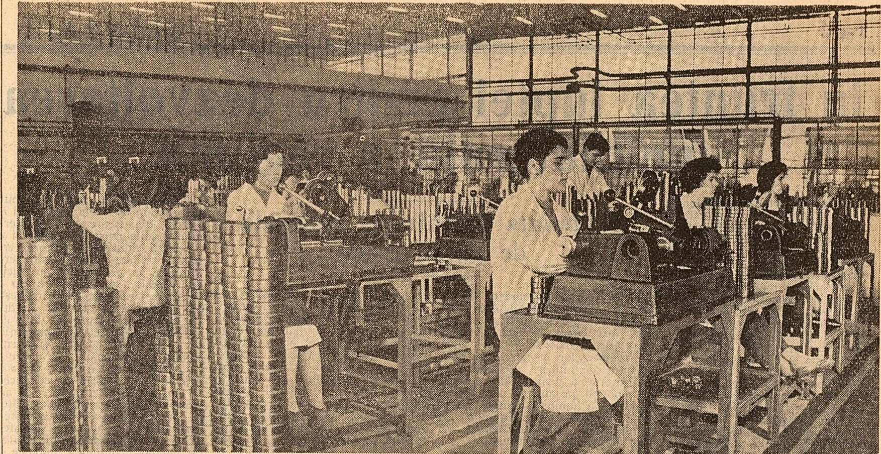
In secția control tehnic de calitate de la uzinele „Rulmentul”-Brașov. (Foto: M. Andreescu)
