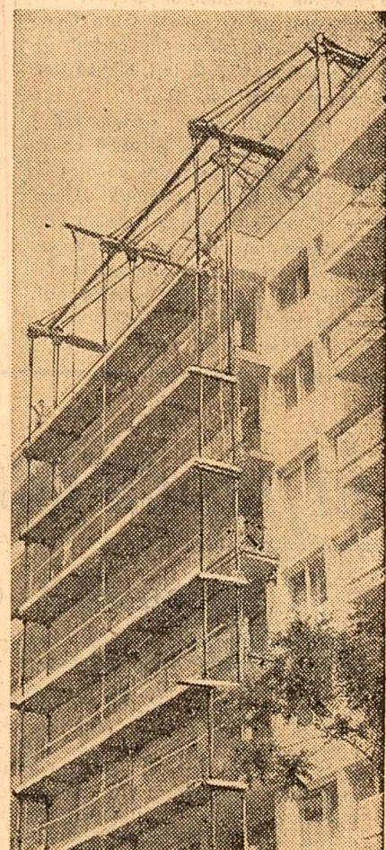
La finalizarea exterioră a blocurilor de locuințe se folosește, pe unele șantiere, un nou tip de schele — schele mobile suspendate. Prin aceasta se economisesc însemnate cantități de material lemnos. În fotografia de astăzi de șchelă montată la blocul D 5 din șoseaua Mihai Bravu din Capitală. (Foto: M. Cloc)
