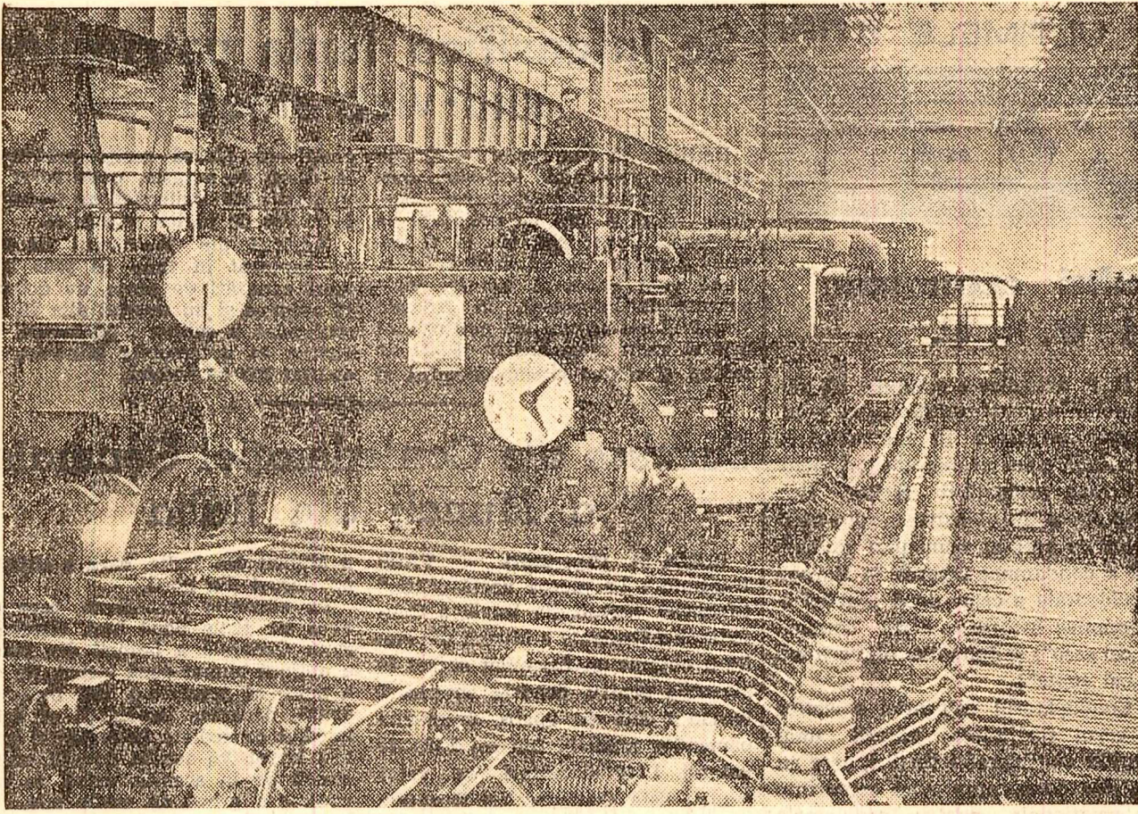
Fabrica de țevi din Roman. Linia de perforare
