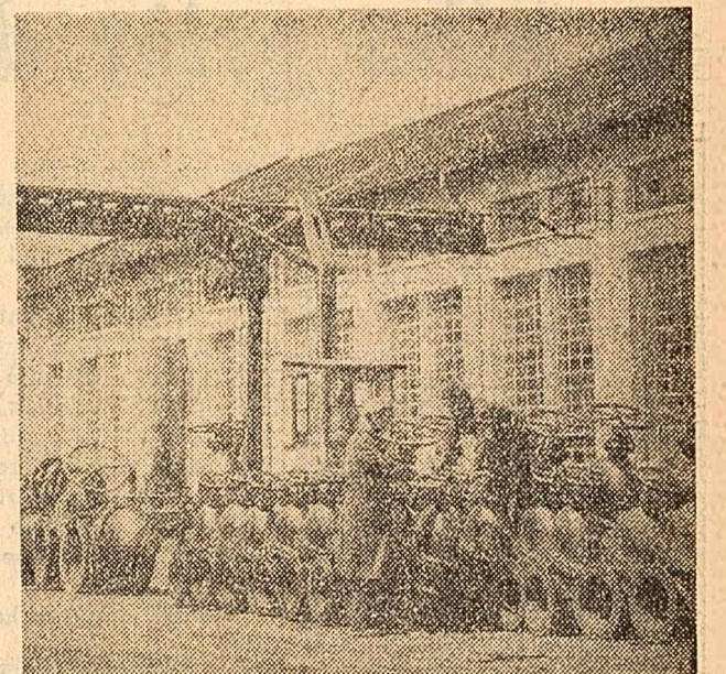
Uzina „Metalurgica” Bacău. Maistrul I. Godea și șeful de echipă J. Cambos fac o ultimă verificare la vamele destinate industriei petrolifere. (Foto: Agerpres)
