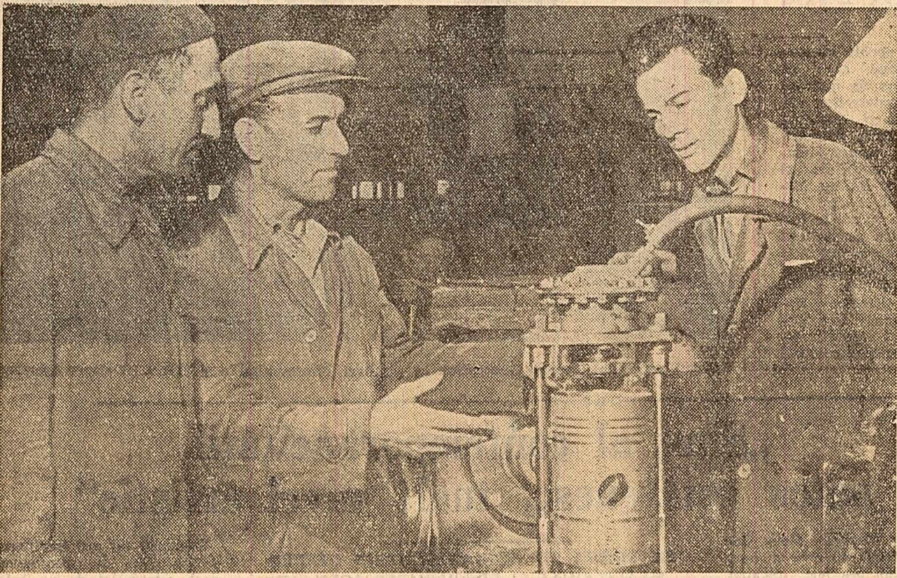
Maistrul Ion Nedelcu, din secția reparării motoarelor a Uzinelor „Poiana”-Cimpina, explică muncitorilor Nicolae Bobiltea (stânga) și Tudor Macău (dreapta) cum funcționează dispozitivul pneumatic pentru prelucrarea pistoanelor adaptat la strunguri în urma propunerilor făcute de muncitori într-o consfățuire de producție.
