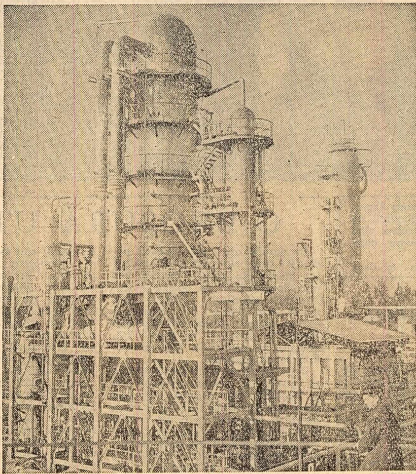
Aspect din secția distilație atmosferică și în vid a țiteiului, de la Rafinăria Cimpina.
