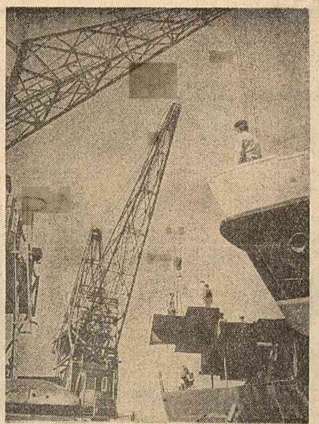
Șantierul Naval Oltenița. Se execută cuplarea punții la o motonavă de 2 000 de tone. (Foto: Agerpres)
