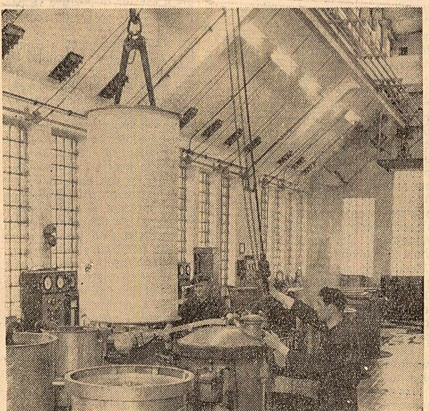
Teșătorii „Răscoala din 1907” din Capitală. Colectivul întreprinderii realizează produse de bună calitate în diferite culori și desene. În fotografie: muncitorul Dumitru Alexandru mamevreață urzeala pentru a fi introdusă în aparatul de vopsit. (Foto: Agerpres)
