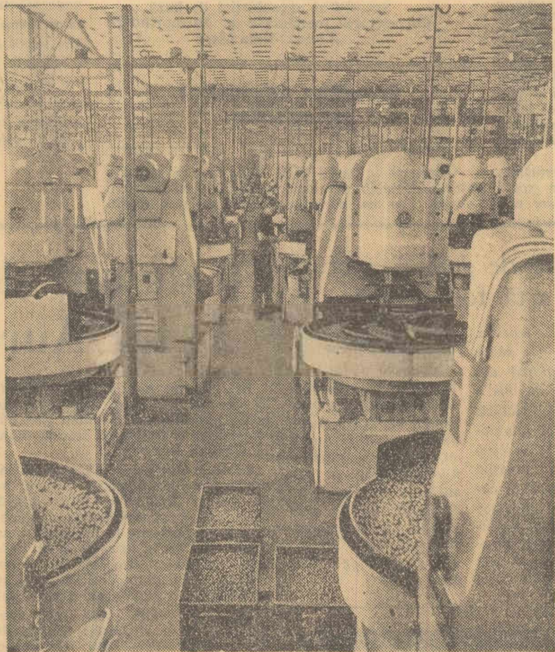
Fabrica Rulmentul din Brașov. În fotografie: aspect din secția în care se produc bilele, secție înzestrată cu mașini moderne, de înaltă tehnicitate.
