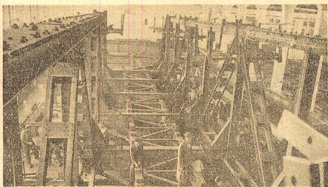
Întreprinderea de poduri metalice și prefabricate din Pitești. Se montează un nou pod.
