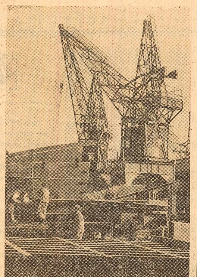
Colectivul Șantierelor navale Oltenița a extins sudura automată față de anul trecut cu 15 la sută. Pe scară tot mai largă este folosită și sudura în mediu de bioxid de carbon. Peste 100 piese metalice pentru instalațiile sanitare interioare de la vase sînt executate din mase plastice. Aici sînt folosite, cu bune rezultate, și unele metode avansate de lucru. Numai montarea pe cala a agregatelor mecanice a dat posibilitate colectivului șantierului să reducă termenul de execuție a unei motonave, în medie, cu 35 de zile. Recent, colectivul șantierului a lansat la apă cel de-al 38-lea vas de 1.000 tone pentru transportul micrcrușilor. În fotografie: Un aspect de pe șantier.
