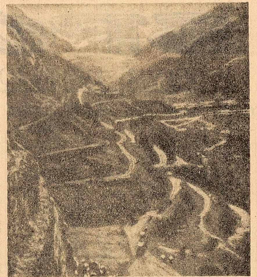
Vedere de pe șantierul hidrocentralei Kaunertal. În această pitorească vale a Tirolului se construiește cea mai mare hidrocentrală cu lac de acumulare din Austria. Ea va furniza anual 570 milioane kilowatt-ora. Primele agregate ale hidrocentralei vor intra în funcțiune în toamna anului 1964.
