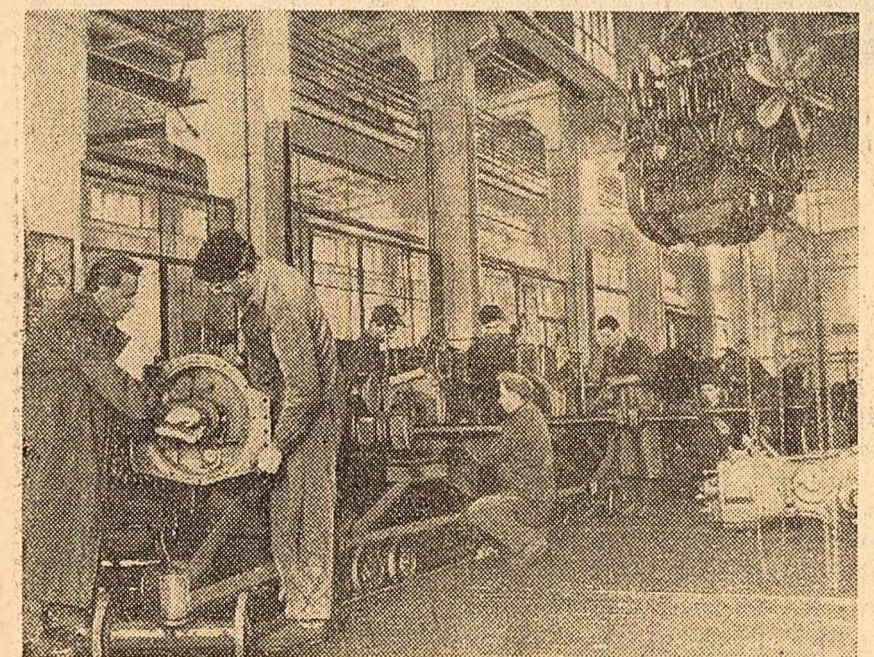
În uzina de reparații Brașov a Consiliului Superior al Agriculturii se lucrează după metoda de flux continuu. Prin aceasta capacitatea de reparații a uzinei s-a dublat, folosîndu-se același spațiu tehnologic. În fotografie — aspect de la montarea pe o linie specială a punților de tractor. (Foto: A. CARTOJAN)
