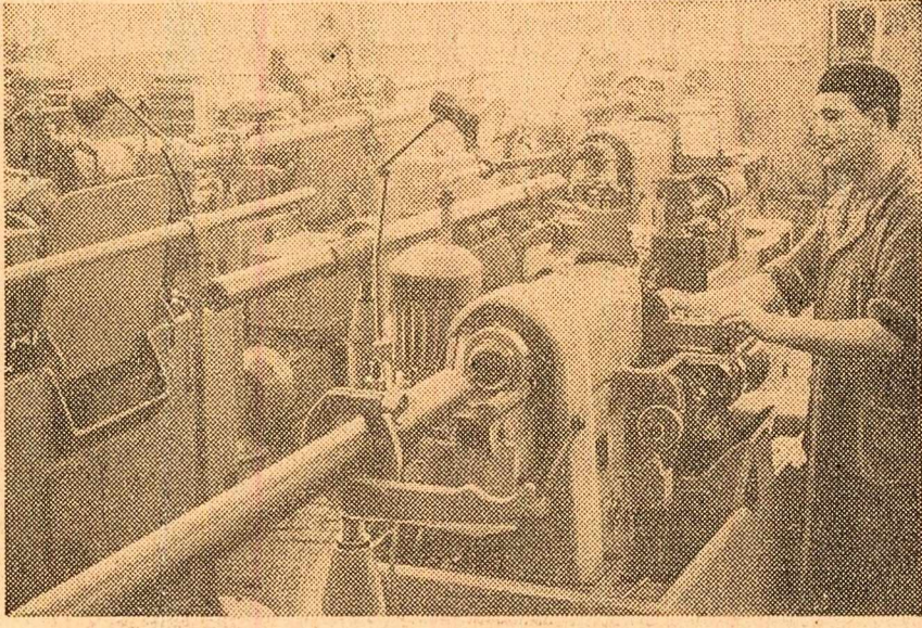
Atelierul de strunguri automate al Uzinei „Electroaparati” din București are prevăzută în planul său pe 1964 fabricarea a peste 100 noi reperi. În vederea executării acestora se iau măsuri pentru reamplasarea mașinilor conform unui flux tehnologic mai rațional care va contribui la sporirea productivității muncii și reducerea timpilor neproductivi ai mașinilor.
