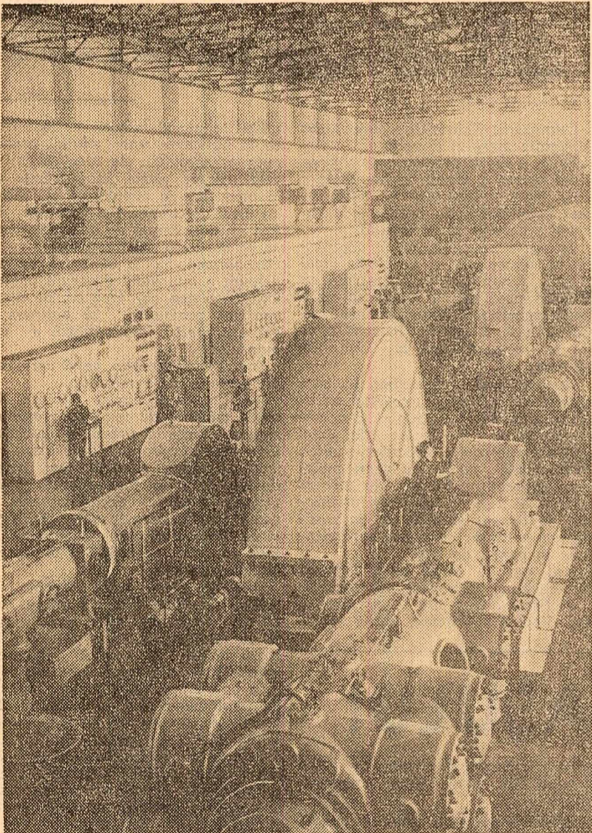
Sala compresoarelor a Combinatului de Ingrășăminte azotoase-Piatra Neamț. Foto: GH. VINTILĂ
