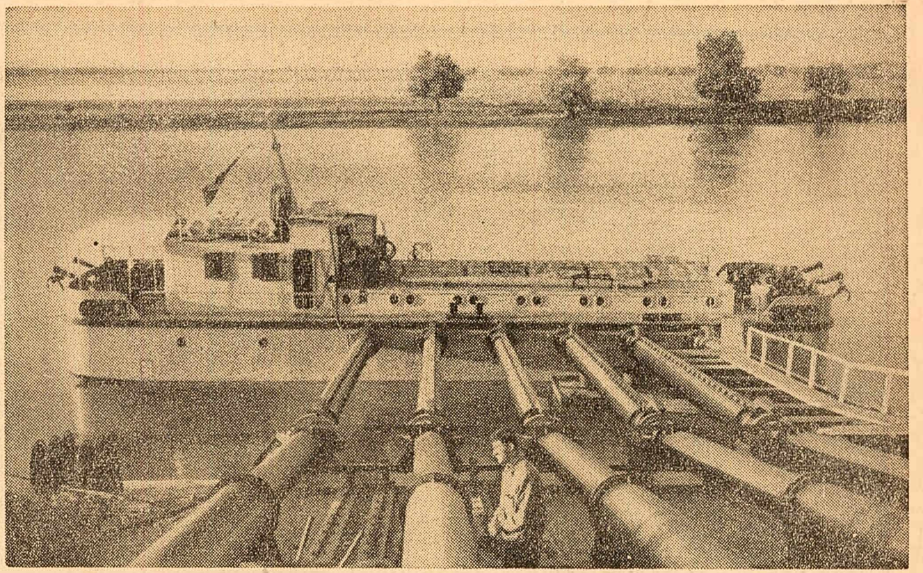
Stație plutitoare de pompare a apei din Dunăre destinată irigațiilor.
