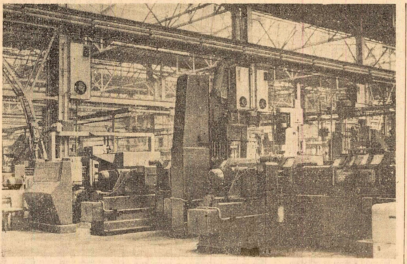
Uzinele „Tractorul” din Brașov. Linia automată de transfer pentru prelucrarea blocului cilindrilor de la tractoarele U-650
