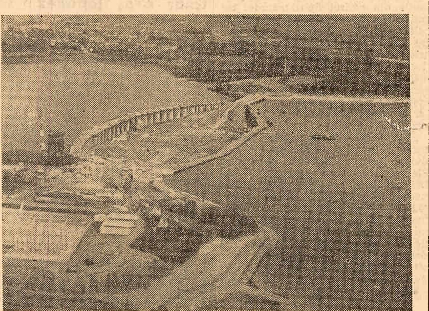
La Ramca, în apropiere de Saint-Malo (Franța), se construiește o uzină mareomotrică (acționată de fluxul mării). Aceasta va fi prima uzină electrică de acest fel din lume
