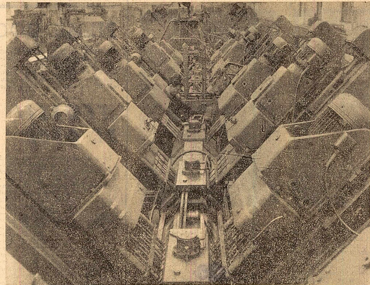
Linie automată de producție la Uzinele „Steagul roșu” din Brașov
