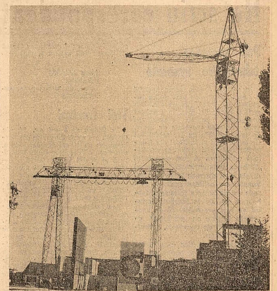
Macaralele turn și capră, de mare tonaj, sînt tot mai des întîlnite pe șantierelor de construcții. Foto: M. Cioabă
