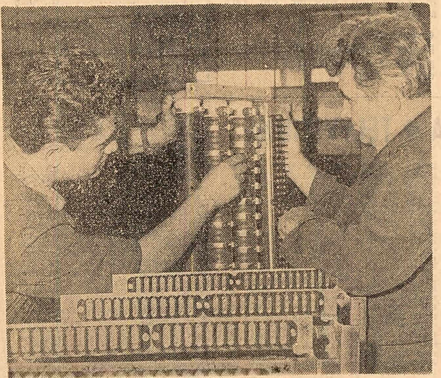
Oameni cu inițială și înaltă calificare, maeștrii Ion Arghiroiu și monștorul Toma Ionă, de la întreprinderea „Electrotehnică” din Capitală, cu găsii noi posibilități de îmbunătățire a calității unor rezistențe pentru locomotivele Diesel-eletrice
