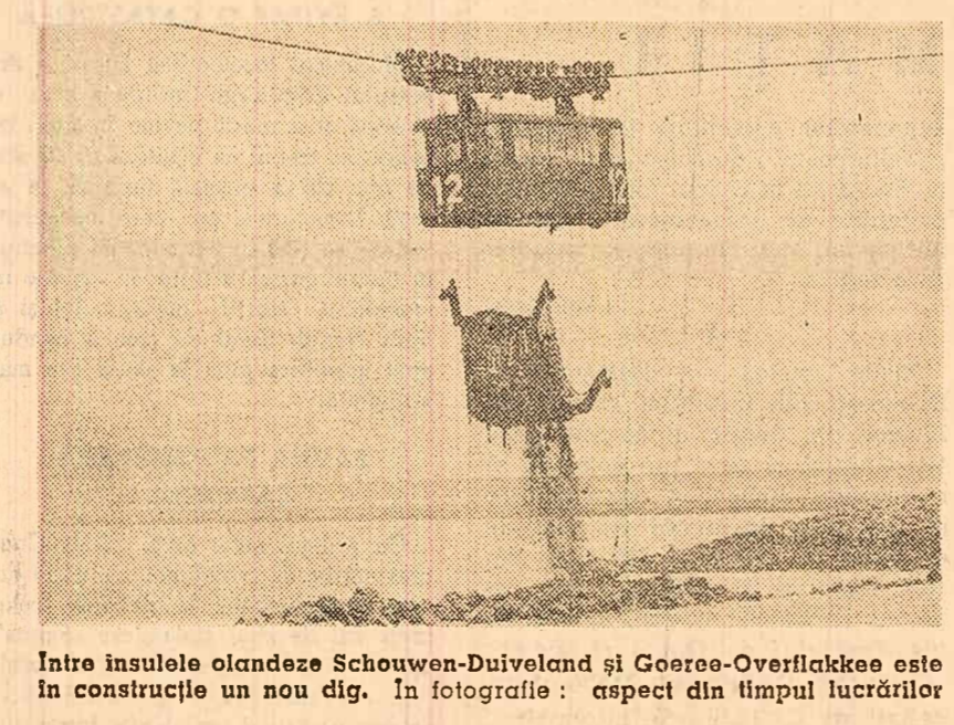
Intre insulele olandeze Schouwen-Duiveland și Goeree-Oversluis este în construcție un nou dig. În fotografie: aspect din timpul lucrărilor
