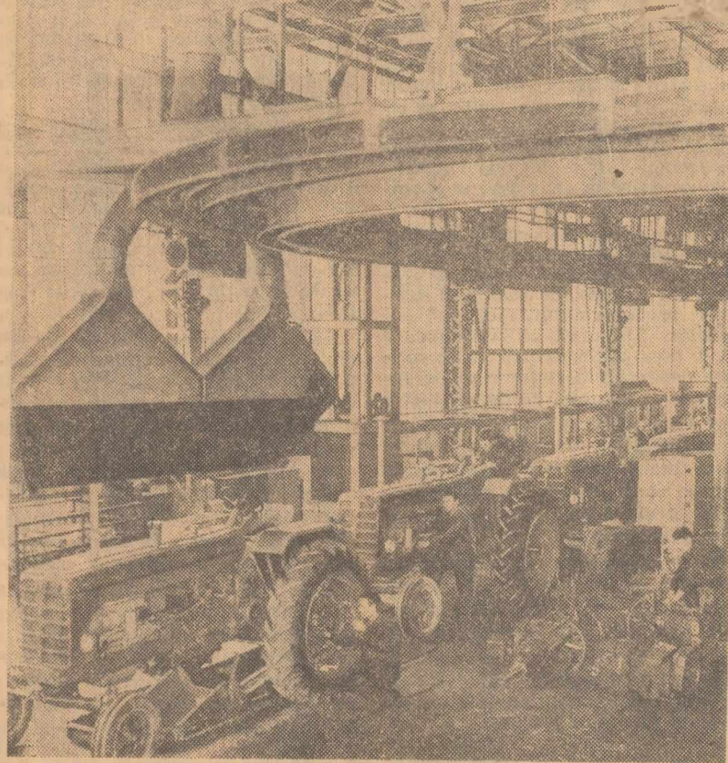
Haia de montaj final a Uzinelor „Tractorul”-Brașov Foto: R. Costin
