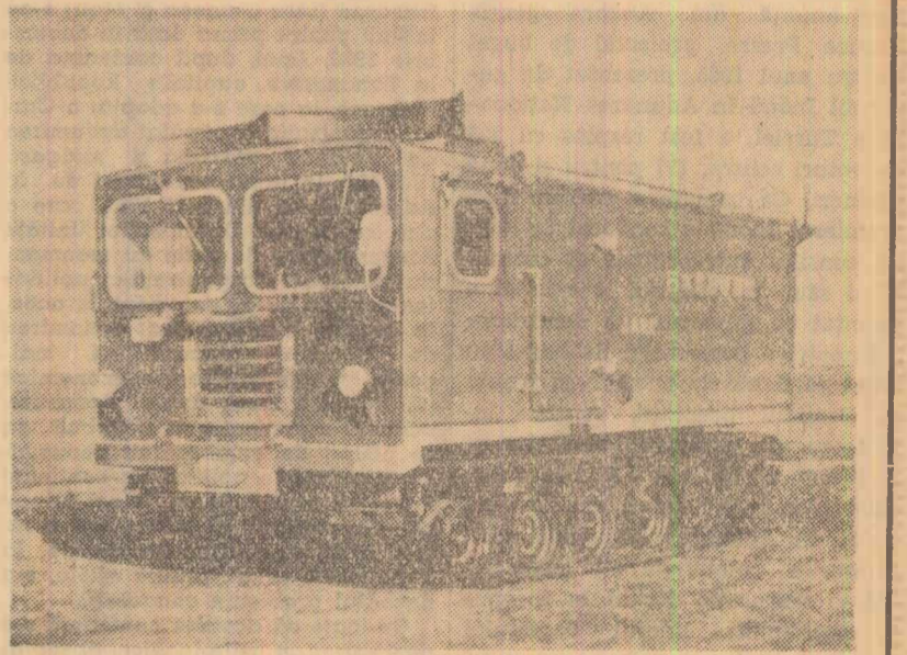
Un nou vehicul pe șenile construit la Tokyo. El va fi folosit în expediția din Antarctica din luna noiembrie 1965. Vehiculul, care se aseamănă cu o locomotivă, are o rază de acțiune de 6.000 km și poate lucra chiar și la o temperatură de minus 60° C
