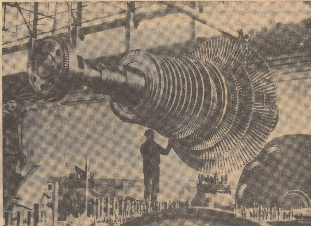
Pe șantierul central electric de termoficare București-Sud, lucrările de construcții-montaj se desfășoară în ritm susținut. În fotografie: Se montează rotorul turbinei nr. 1 de 50 MW
