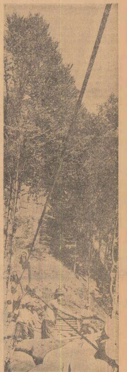
La punctul terminus al funicularului exploatarea forestieră Vizanca (I.F.E.T. Vrancea, regiunea Galați)
