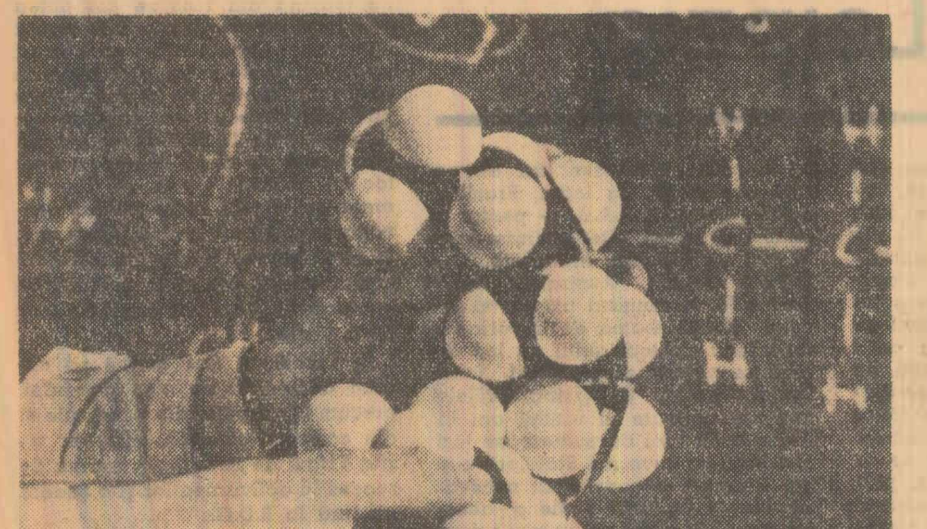
Moleculele, oricît de mari ar fi, nu pot fi zărite cu ochiul liber. Mijloacele moderne de cercetare permit însă realizarea unor modele — mult mărite — care oglindesc structura și contribuie la înțelegerea proprietăților lor
