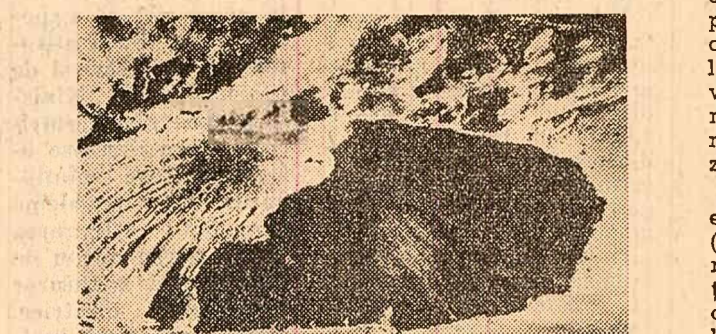
Craterul meteoric din Arizona (S.U.A.)
