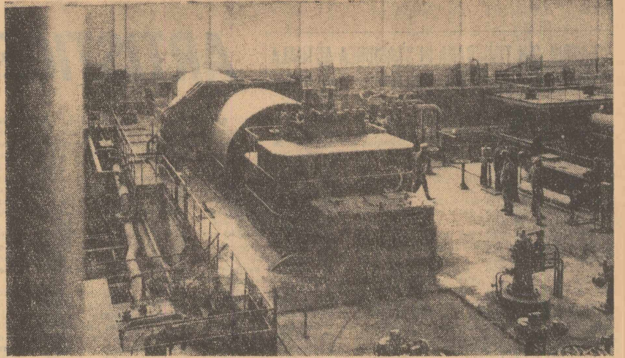
La centrala electrică de termoficare București-sud a intrat în funcțiune, cu cîteva zile mai devreme față de termenul prevăzut în grafic, cel de-al doilea grup turboagregator de 50 MW. În prezent, constructorii electricitii lucrează pentru extinderea centralei cu încă două agregate de cîte 100 MW. În fotografie: una din turbinele de 50 MW
