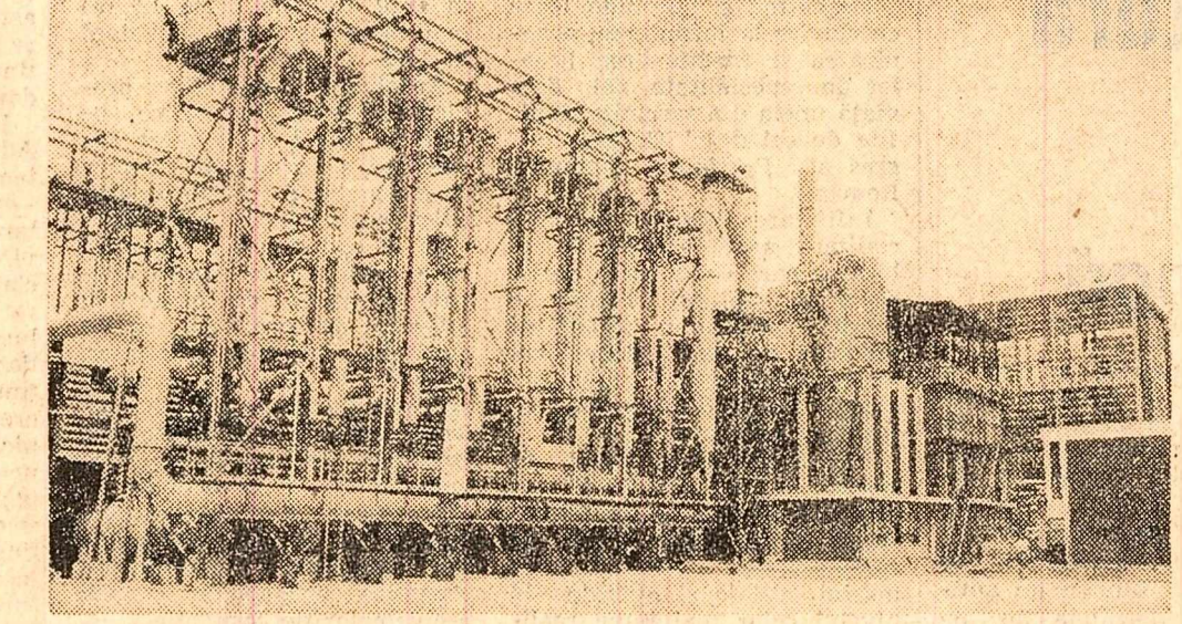
Instalații ale Uzinei de negru de fum din Pitești, a cărei construcție se apropie de sfîrșit. Foto: Gb. Vintilă
