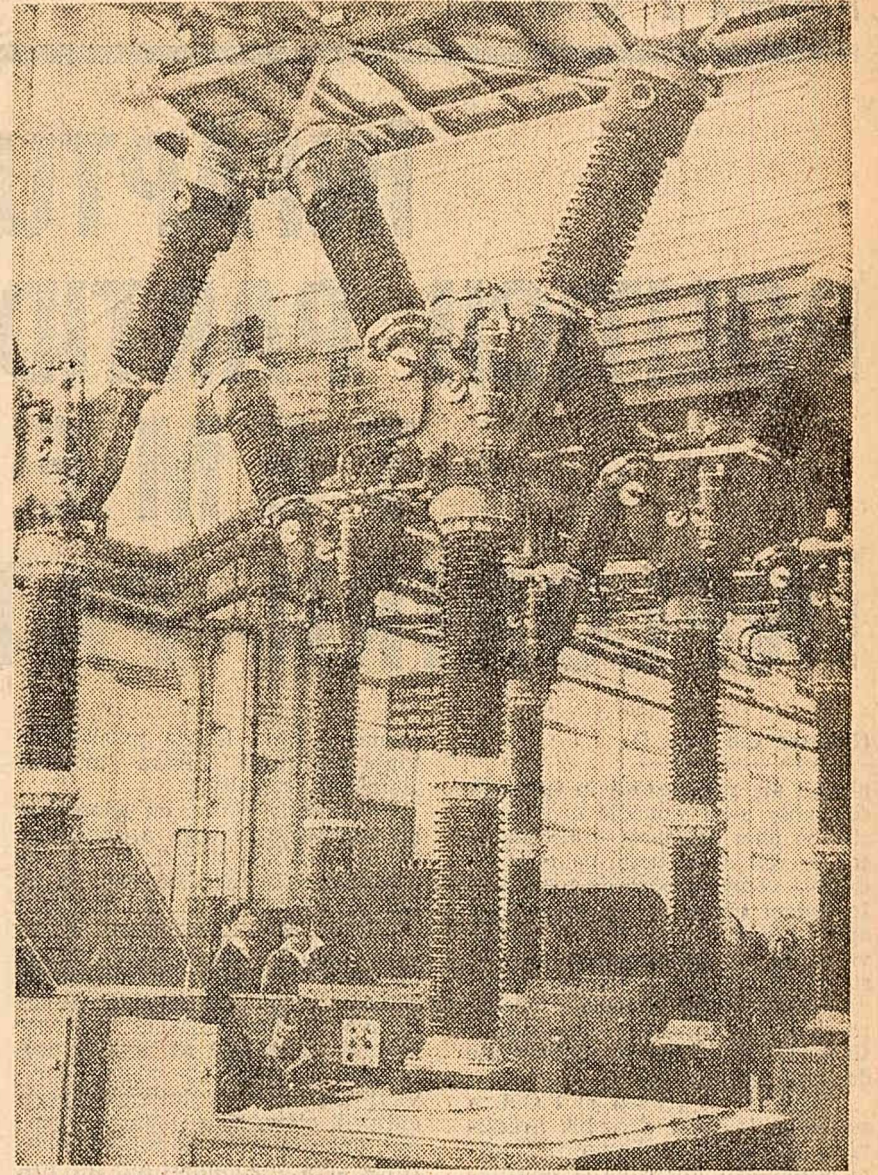
Uzinele „Electroputere” din Craiova: Întrepruători de 220 kw realizați în noua hală a fabricii de mașini electrice rotative Foto: Gh. Vinții
