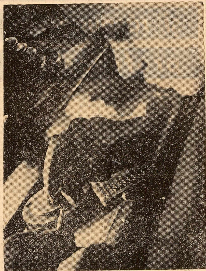
Întreprinderea de piese radio și semiconductori-Băneasa. Închiderea tranzistorilor în atmosferă de aer uscat
