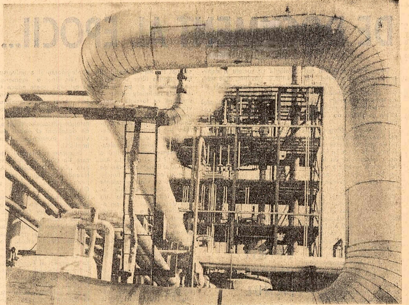
Noua fabrică de anhidridă ftalică, de la Combinatul petrochimic Ploiești Foto: R. Costă
