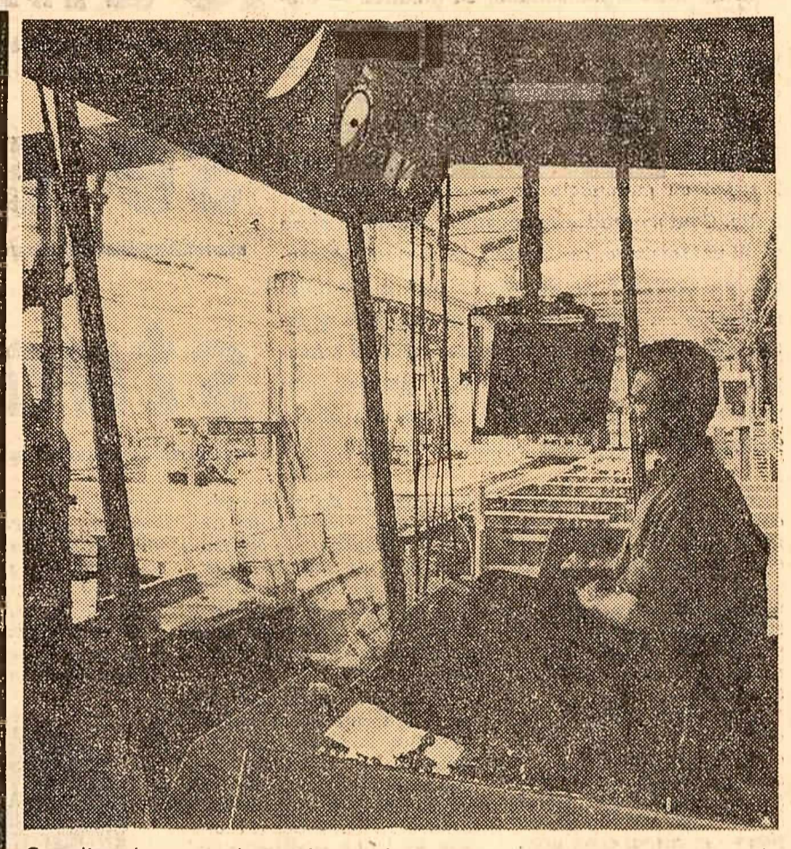
Complicatul proces de producție al laminatului de tablă grosă de la Combinatul siderurgic din Galați este dirijat automat de la cabinele de comandă. (Foto Agerpres)
