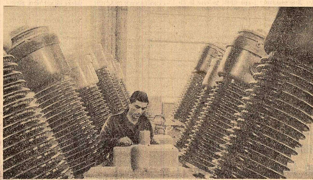
În atelierul interpuțoare de înaltă tensiune de la uzina „Electroputere”-Craiova: se face o ultimă verificare la diferite subsansamble
