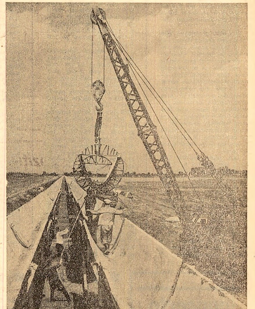
La G.A.S. Dorolj, regiunea Maramureș, se amenajează un sistem modern de irigații pe 2.300 ha, unde apa va fi condusă prin ișchebură de beton. Foto: A. Cartoian
