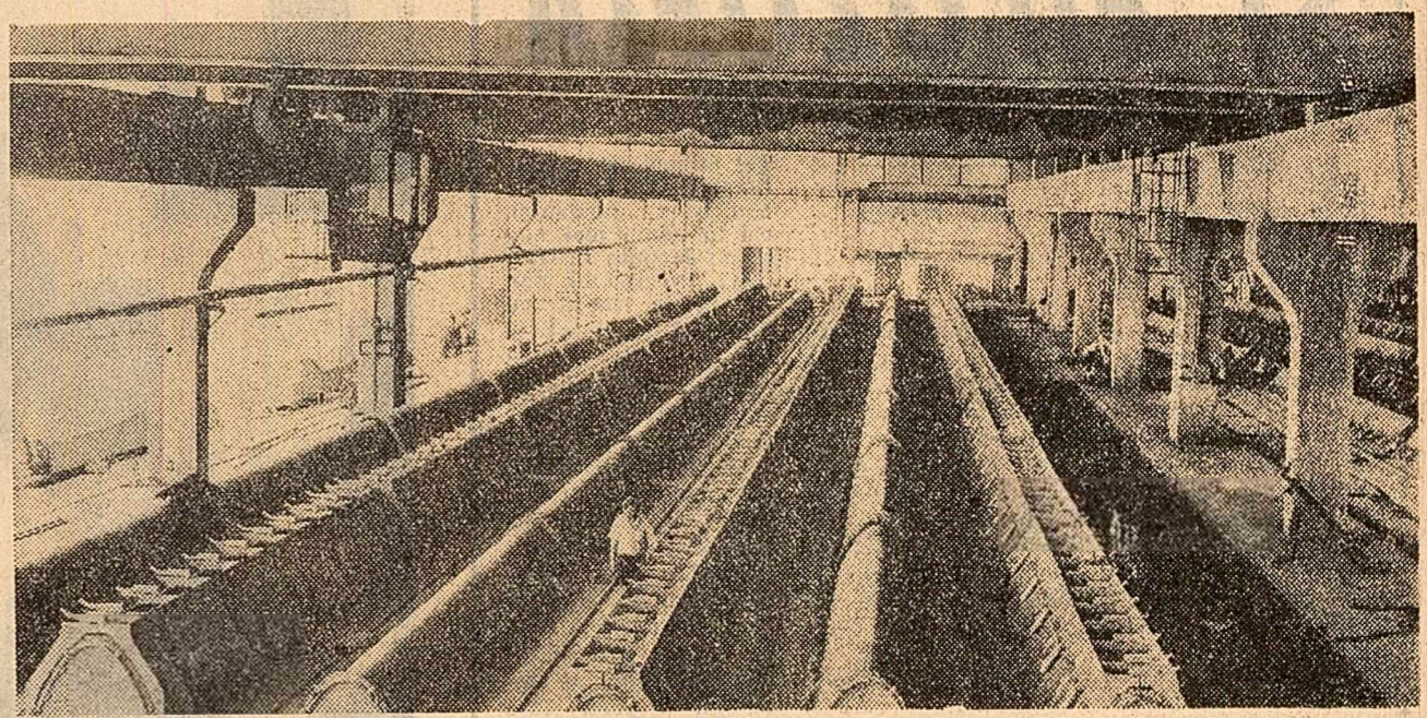
Fabrica de prefabricate din beton Călărași: în secția de elemente din beton armat precomprimat
