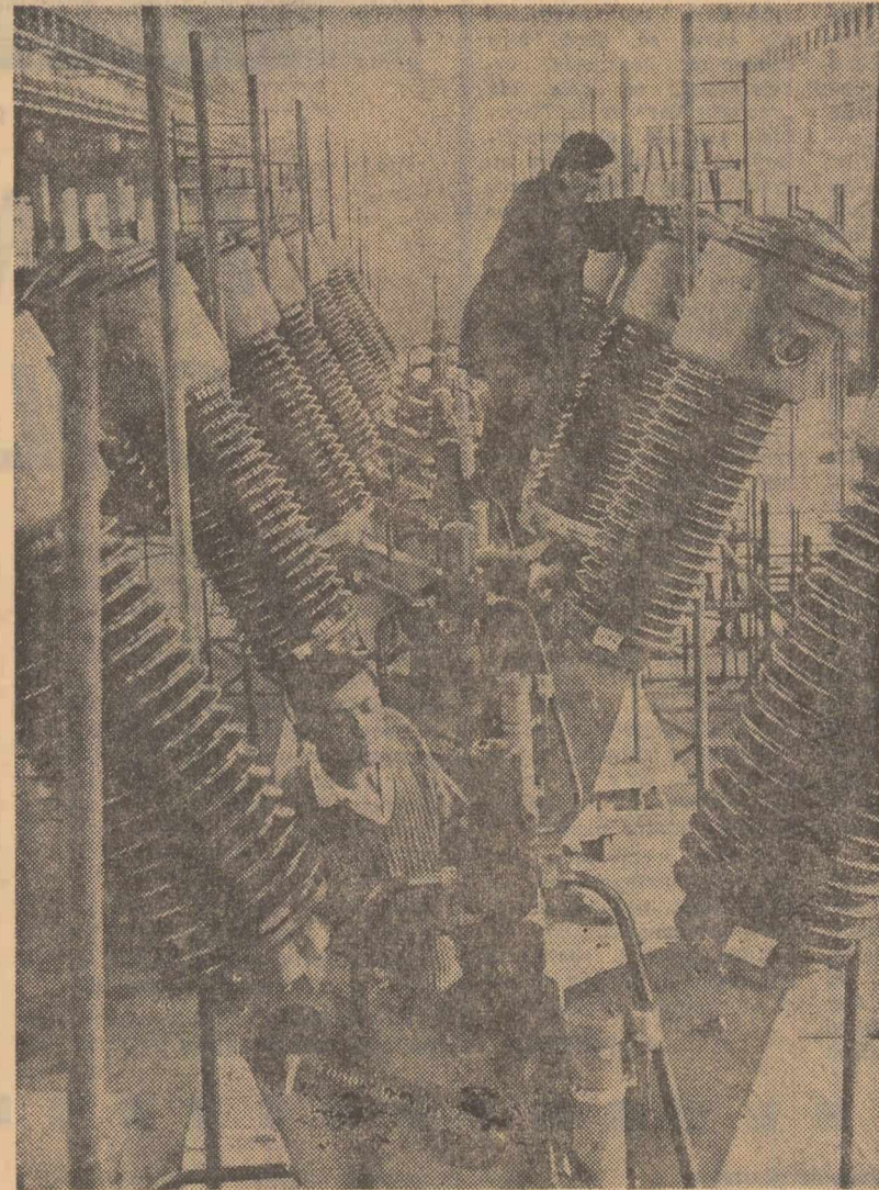
In secția aparatelor a Uzinei „Electropulare”-Craiova: Se verifică un nou lot de interupătoare automate
