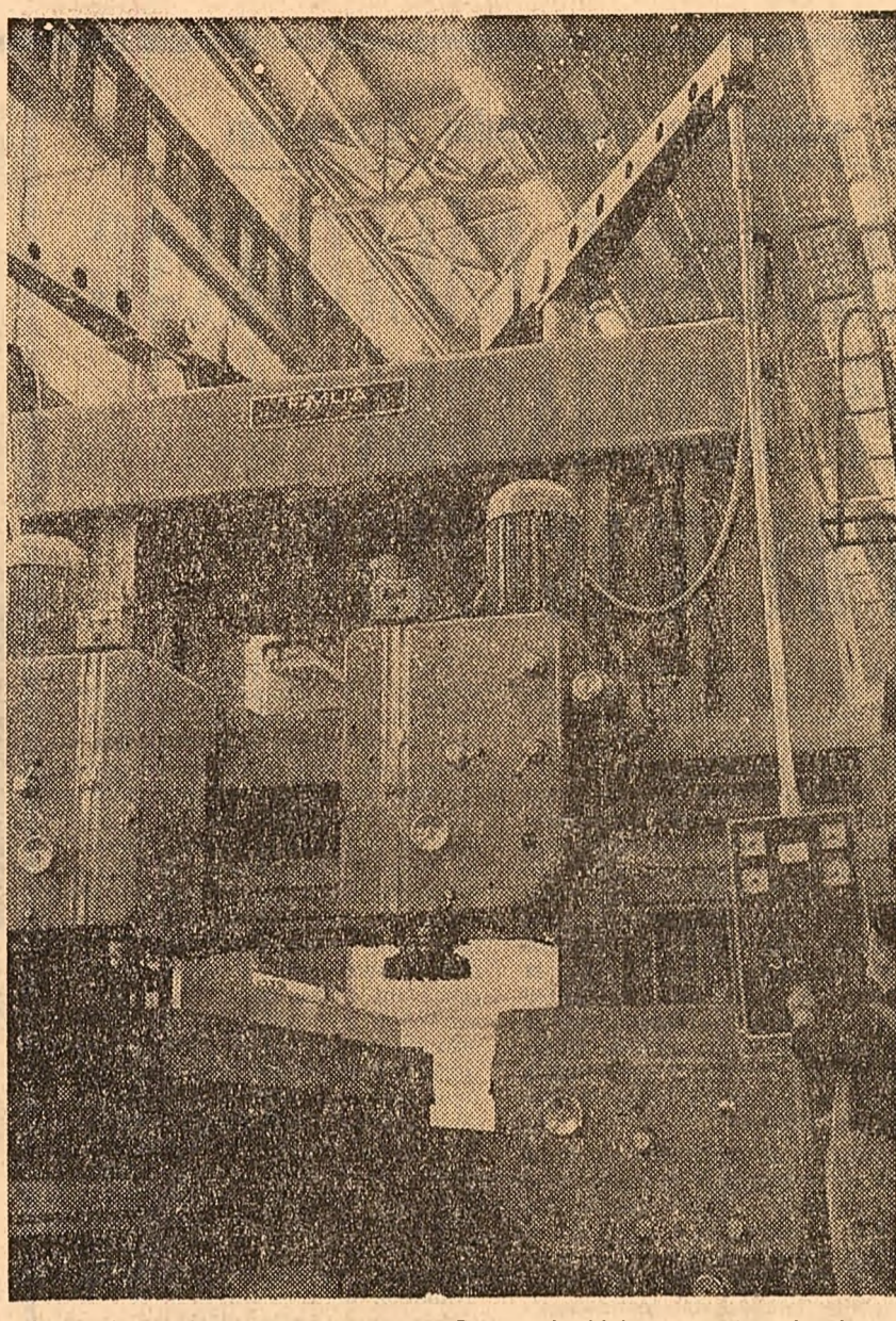
Fabrica de mașini-unelte și agregate București. Aici se produc tipuri moderne de strunguri carusel, mașini orizontale de alezat și frezat. În fotografie: primul exemplar din seria zero a mașinii de frezat longitudinală cu portal — F.L.P.-1 600 Foto: M. Cloș
