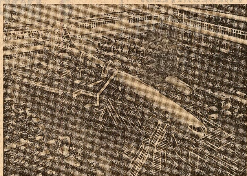
La șantierele Filton, lângă Bristol, continuă construcția variantei „Concorde 002”. Luni, ministrul britanic al tehnologiei a declarat în Camera Comunelor că producția în serie a supersonicului pentru pasageri nu va suferi întârzieri în urma amănunțit impuse zborului inaugural al prototipului realizat în Franța
